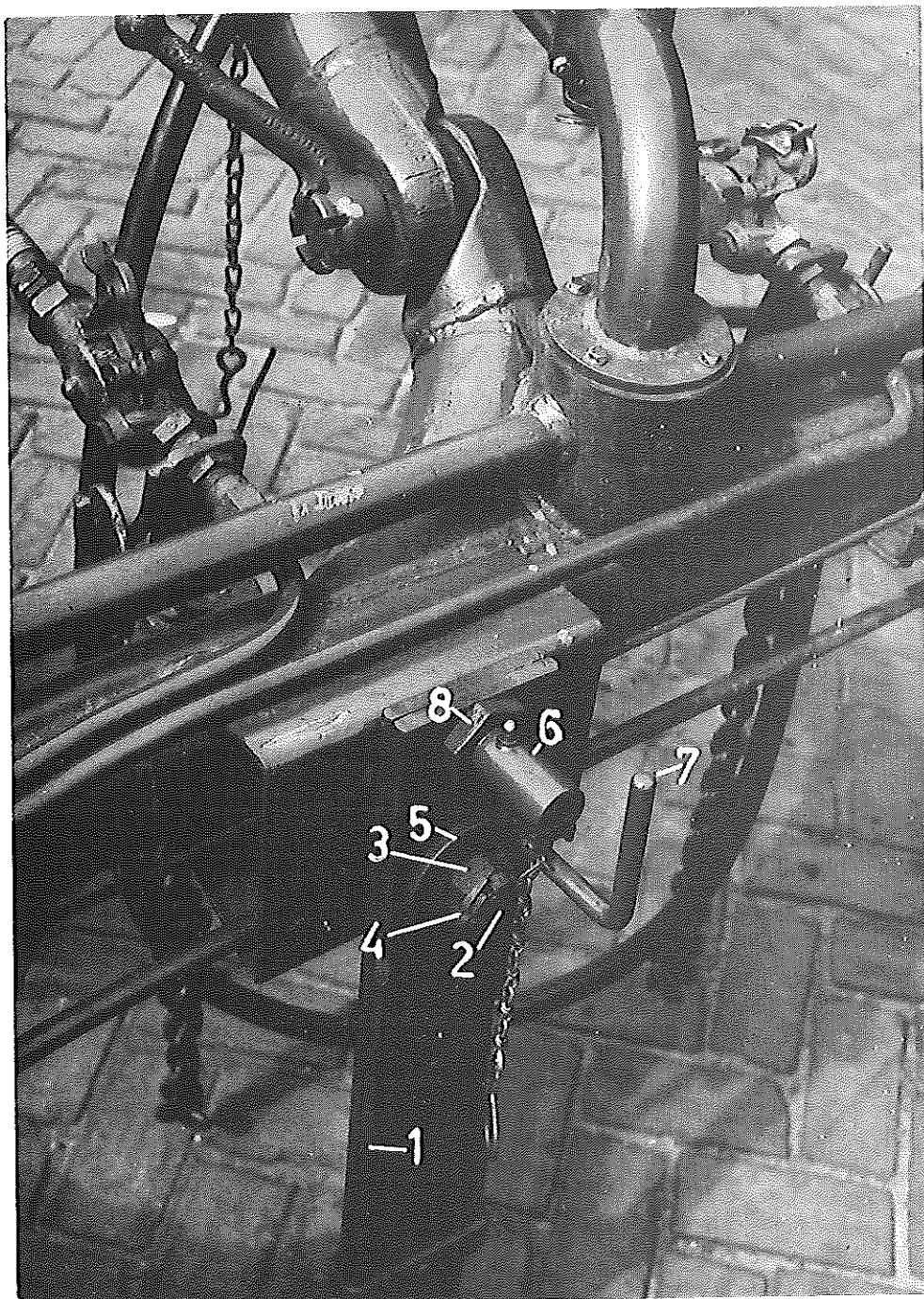
AFB. 37. PARKEERSTEUN VOOR
