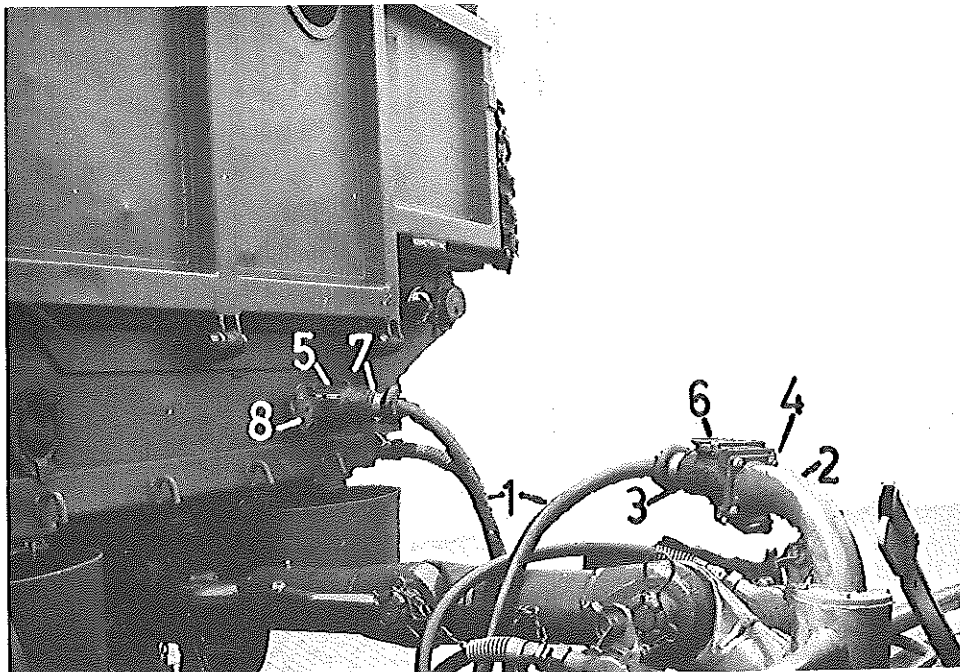
AFB. 39 ELECTRISCHE KOPPELKABEL
