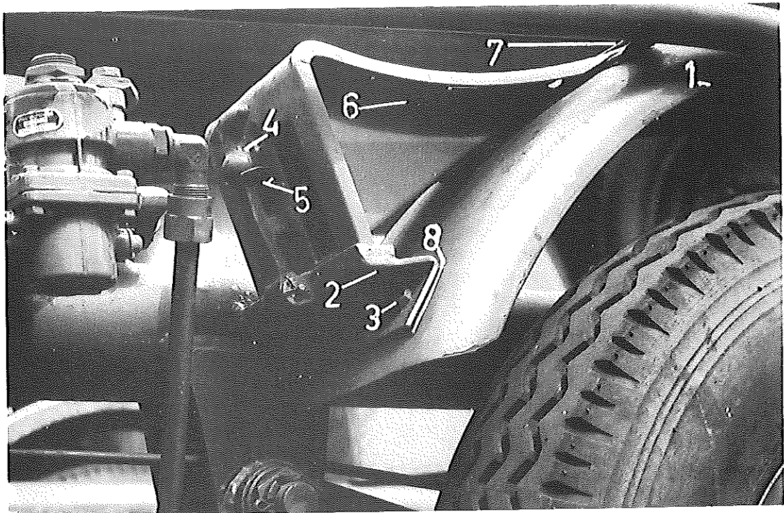
AFB. 33. BEVESTIGINGSSPATSCHERM m/STOPBLOK
